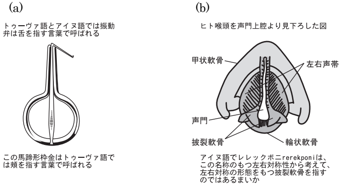
図 11 鉄口琴の図(a)ヒト喉頭を声門上腔から見下した図(b)
