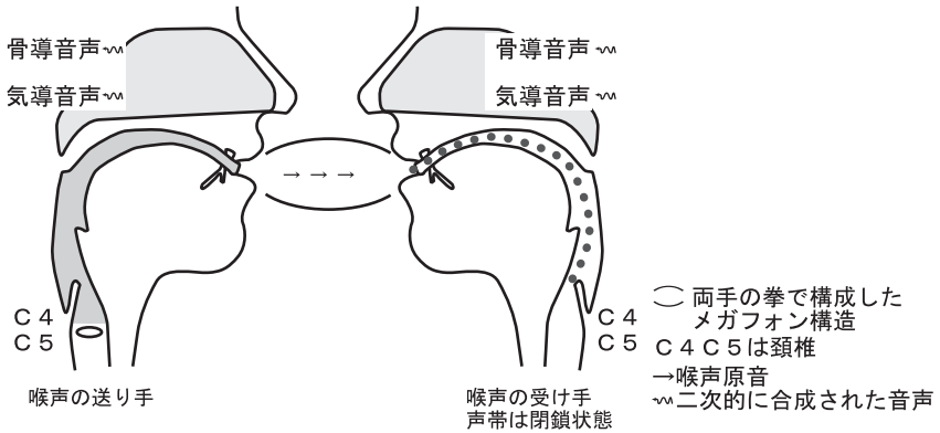
図1 レクッカラの実行概念図：声帯を閉じた受け手が、口腔に送り込まれた送り手の喉声を、無言調音運動によって変調するとき、喉声原音は時々刻々音韻連鎖へと変換される。
