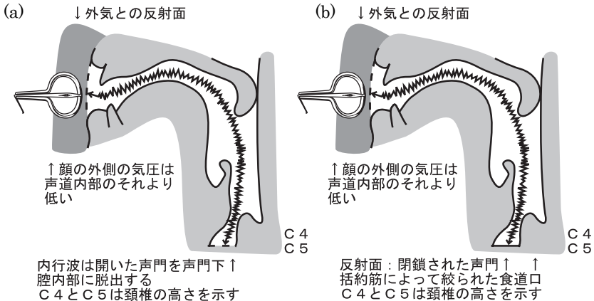
図 8 開管声道での口琴原音の挙動 (a)と閉管声道での口琴原音の挙動 (b):原音への音韻付与は(b)でのみ実現する
