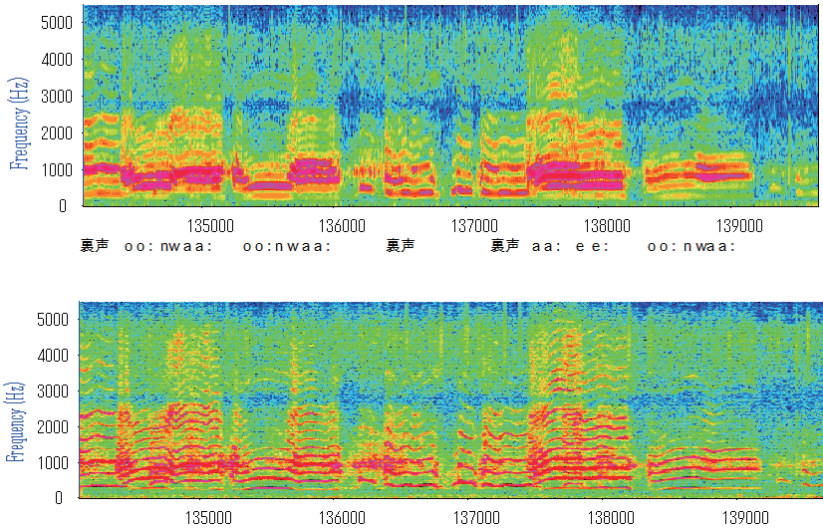
図 25 樺太・栄浜のレクッカラ Type 6 の分析結果：広帯域分析ソノグラム(上)と狭帯域分析ソノグラム(下)
