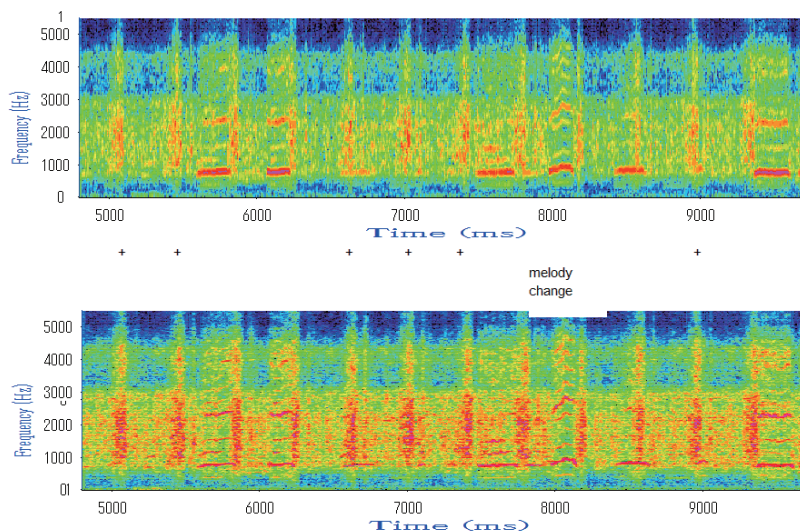
図 17 鳥の鳴き声を真似たと思われる部分の分析結果：広帯域分析ソノグラム（上）；狭帯域分析ソノグラム（下）。
