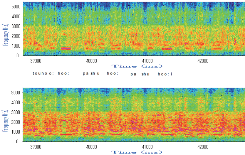
図 16 “ touhoo hoo pashuhoo pashuhoo ”と聞き取られる部分のソノグラム： 広帯域分析ソノグラム(上)；狭帯域分析ソノグラム(下)
