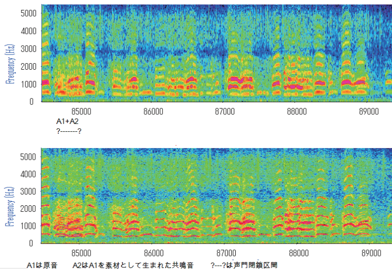
図 23 樺太・栄浜のレクッカラ Type 4 の分析結果：広帯域分析ソノグラム(上)と狭帯域分析ソノグラム(下)。A1 は入力原音、A2 は二次的の共鳴音である。‘?---?’ はソノグラムで確認される有効な閉管(closed pipe)の区間である。
