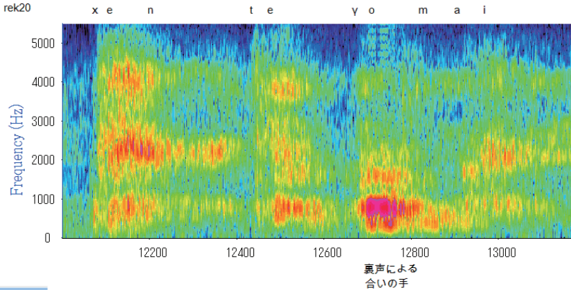
図 27 ピッチエイネンの分析結果：音声表記は筆者(下村)の聞き取りによる推定
