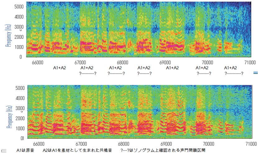
図 22 権太・栄浜のレクッカラ Type 3 の分析結果：広帯域分析ソノグラム(上)と狭帯域分析ソノグラム(下)。A1 は入力原音、A2 は二次的共鳴音である。‘?---?’ はソノグラムで確認される有効な閉管(closed pipe)の区間である。
