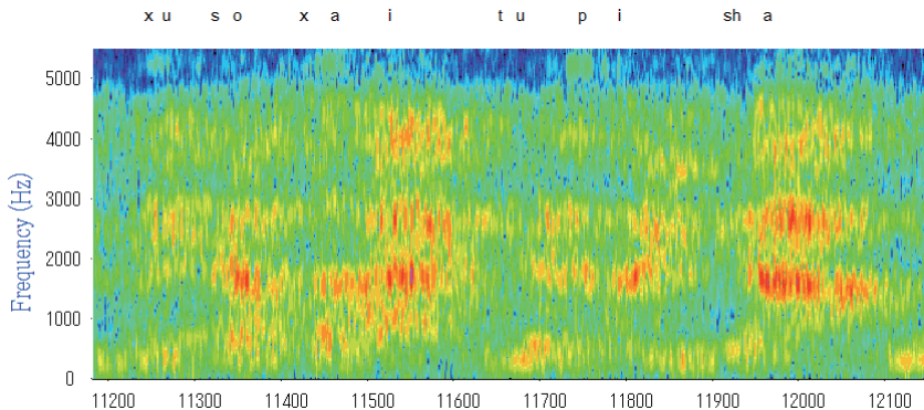
図 26 カタジャックの分析結果：音声表記は筆者(下村)の聞き取りによる推定
